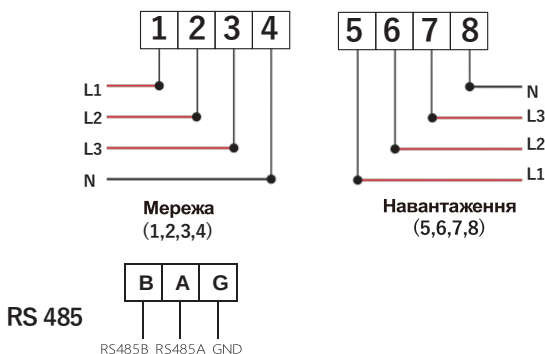
Малюнок 7.18 Лічильник Eastron
