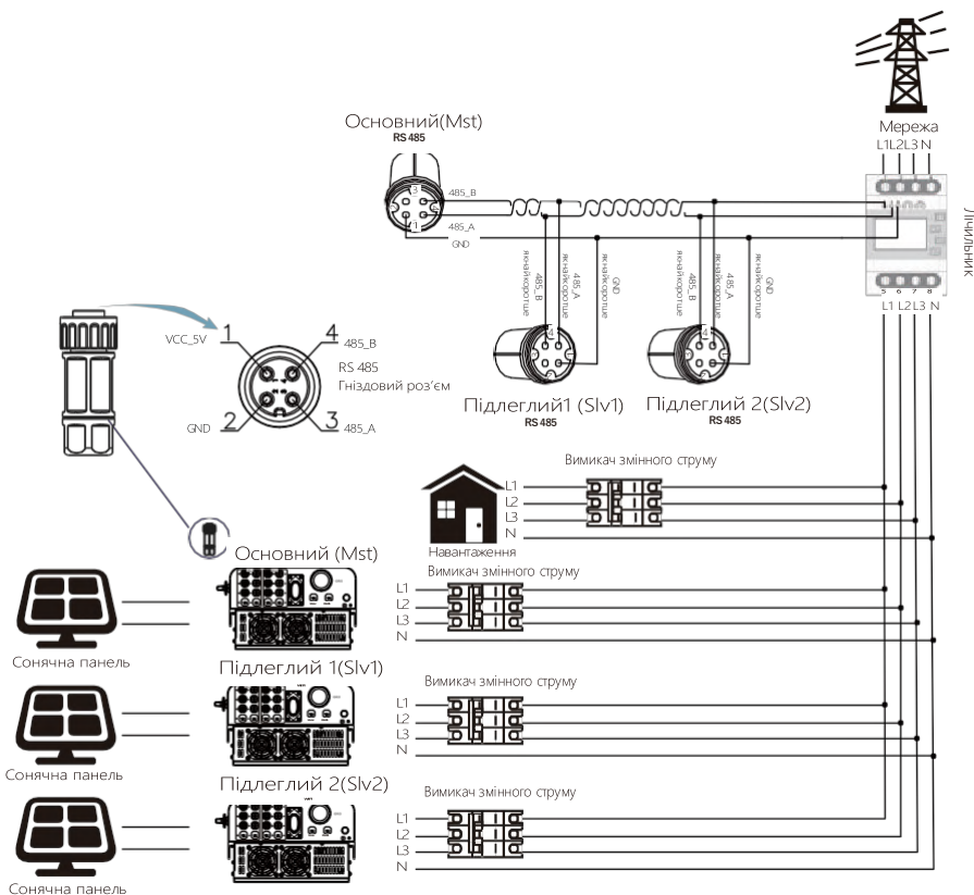
Малюнок 7.19 Схема підключення Eastron (схема проходних каналів)
