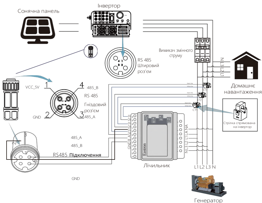
Малюнок 7.8 Схема підключення лічильника Easton
