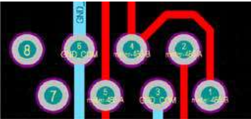
Порт лічильника
