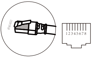
Порт RS485
