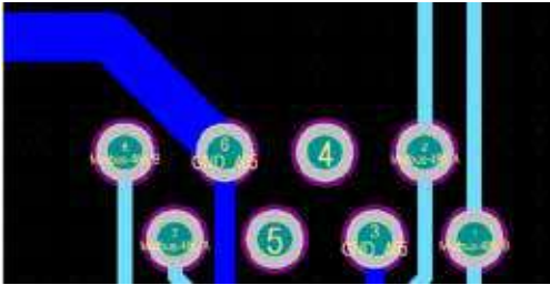
Порт RS485
