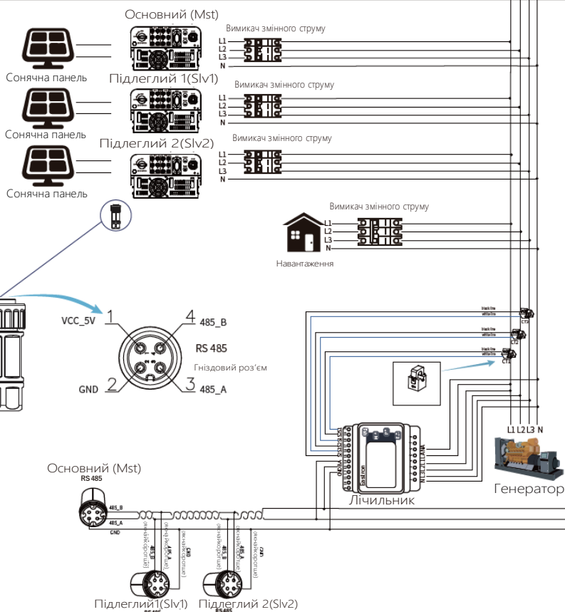
Малюнок 7.25 Схема підключення (трифазна електрика)
