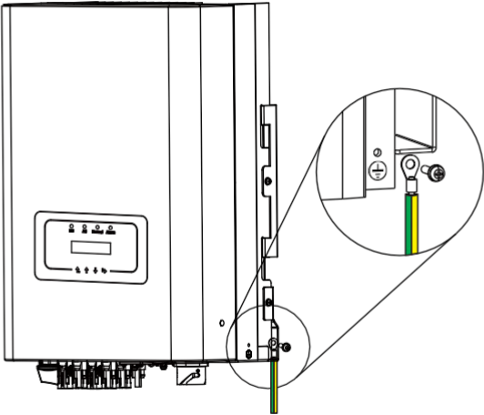
Малюнок 5.11 Встановлення дроту заземлення
