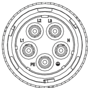
Малюнок 5.9 Схема отворів для роз'єму змінного струму
