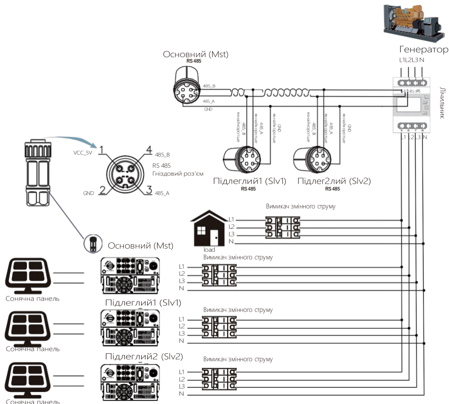
Малюнок 7.21 Схема підключення Eastron (схема проходних)
