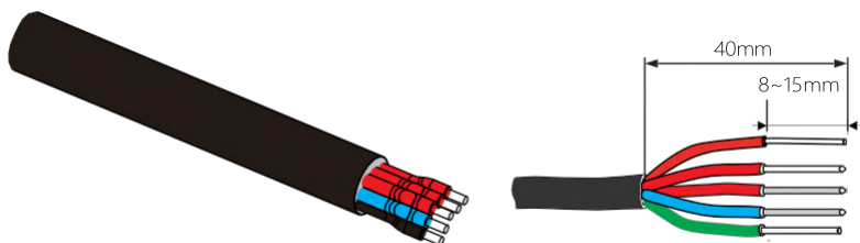
Рис 5.8 Strip AC cable
