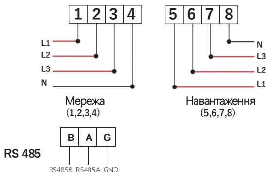
Малюнок 7.20 Лічильник Eastron
