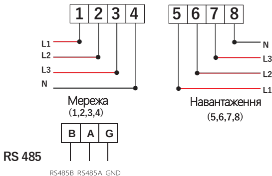
Малюнок 7.1 Лічильник Eastron
