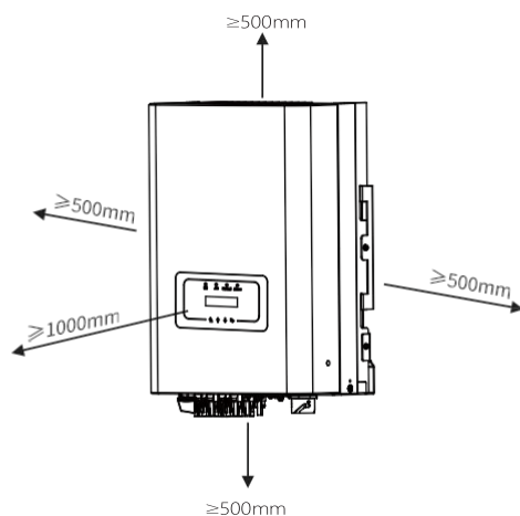
Малюнок 4.3 Проміжок у встановленні
