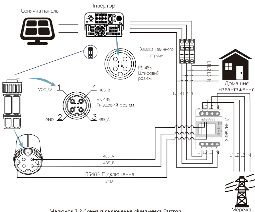
Малюнок 7.2 Схема підключення лічильника Eastron
