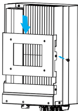
Малюнок 4.6 Монтаж інвертора
