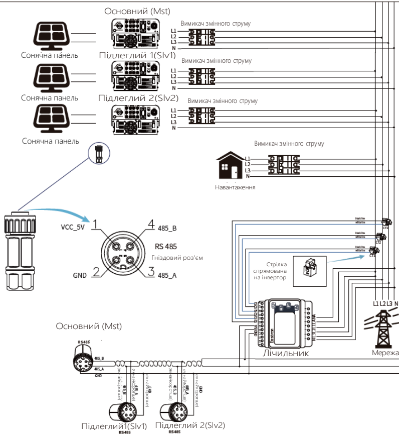
Малюнок 7.23 Схема підключення (Трифазна електрика)
