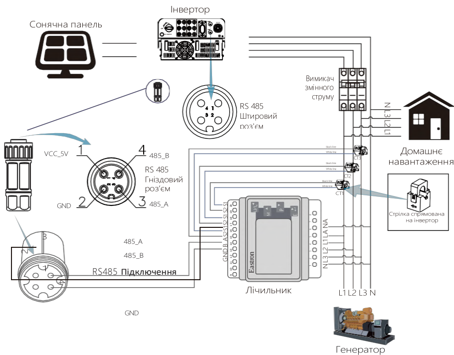
Малюнок 7.8 Схема підключення лічильника Eastron
