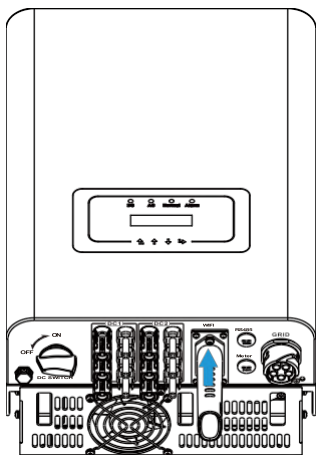
Малюнок 5.13 Схема встановлення реєстратора даних
