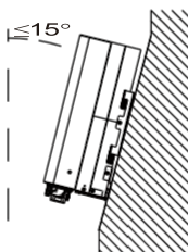
Малюнок 4.2 Кут встановлення
