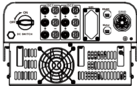
Малюнок 1.2 Вид знизу
